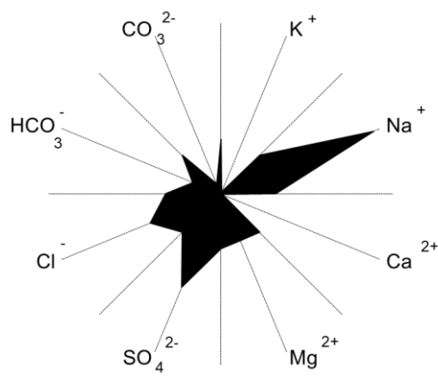
Соленый тип, TDS=6 г/л (Алаколь; № 32.)
