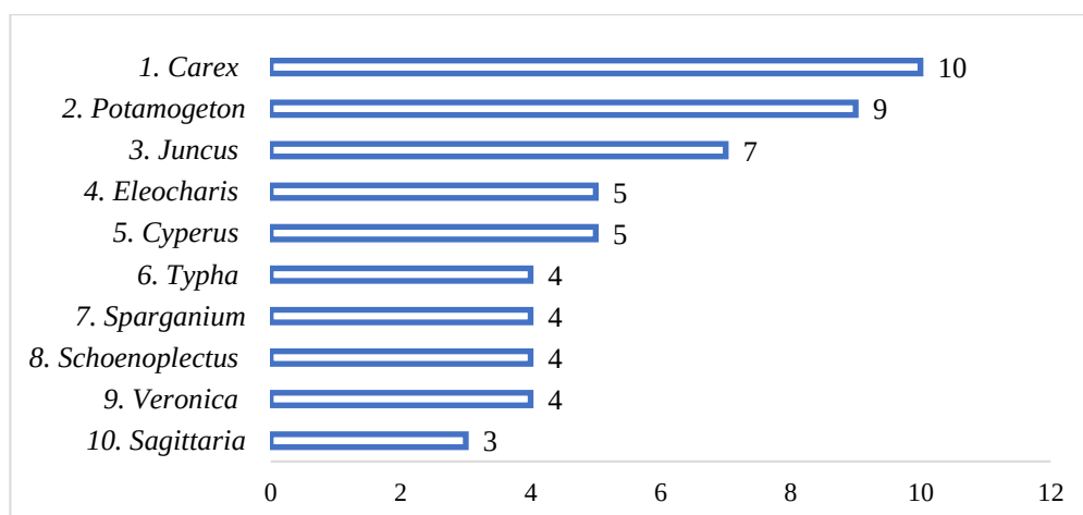
Рисунок 31 – Количество видов для наиболее крупных родов высших водных растений
