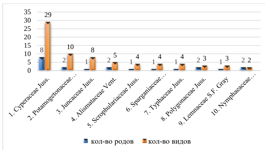
Рисунок 30 - Число видов и родов в 10 ведущих семействах высших водных растений
