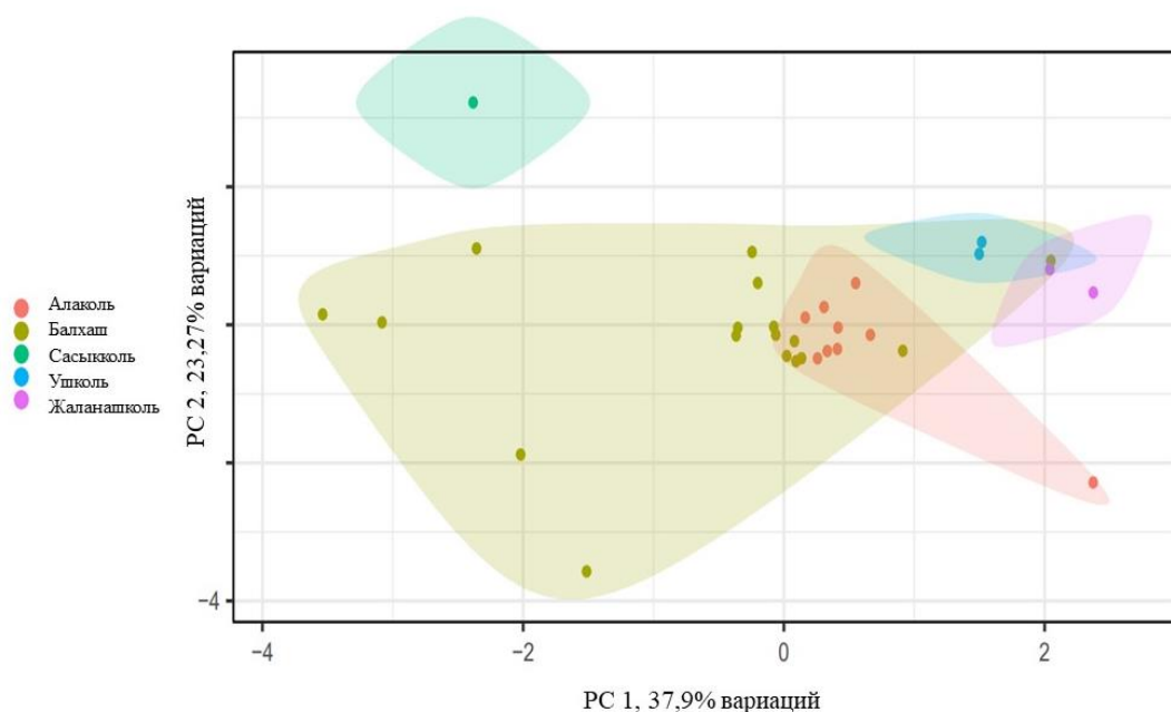
Рисунок 15 - РСА анализ классификации водоемов по приуроченности к местообитанию
