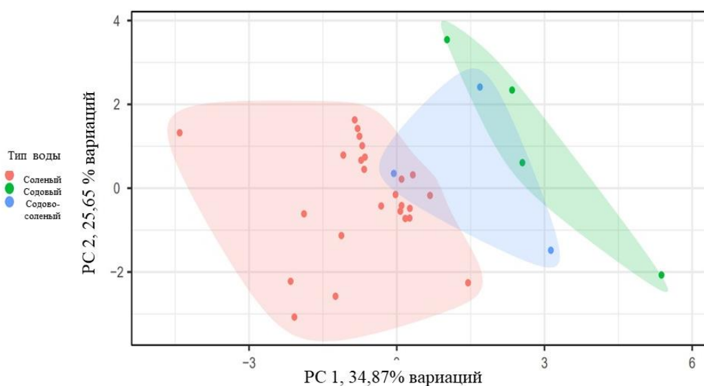
Рисунок 14 – Анализ главных компонент (РСА) по химическому составу воды на основе ионного состава
