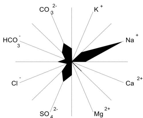
Содовый тип, TDS=2 г/л (Ушколь, № 20)
